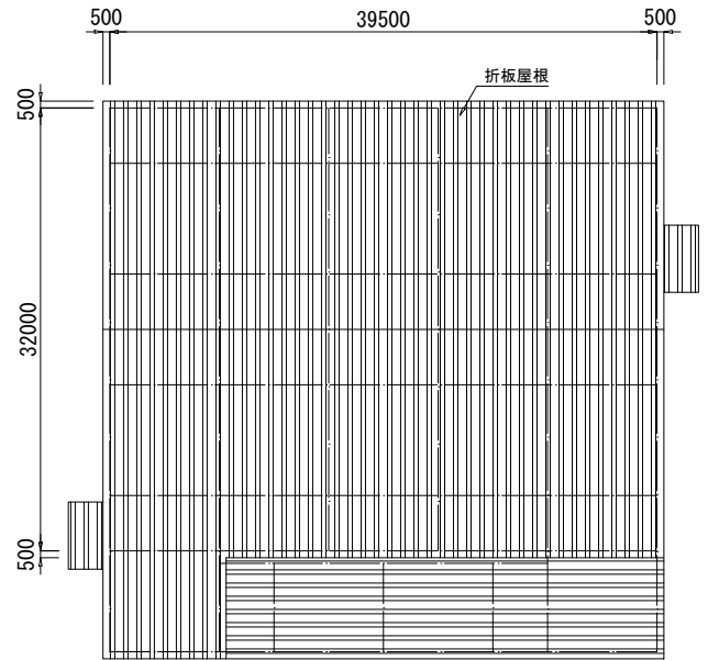
屋根伏図
