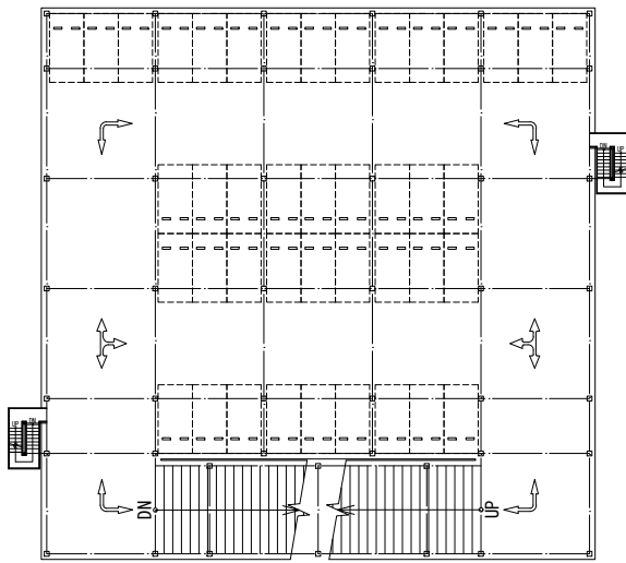
2階平面図
