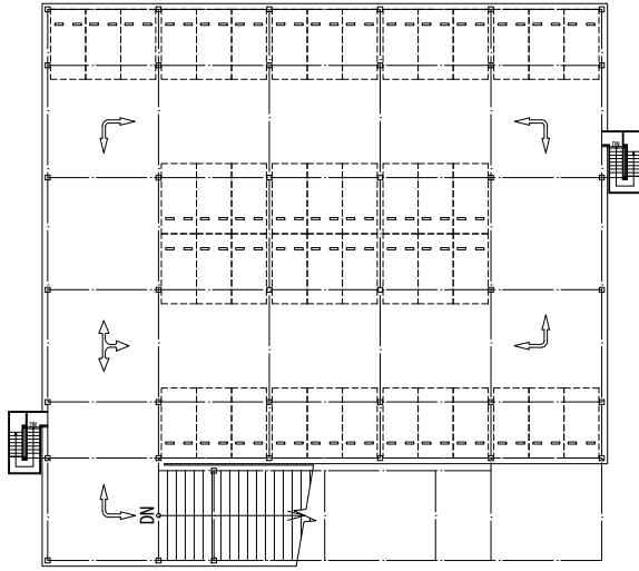
3階平面図
