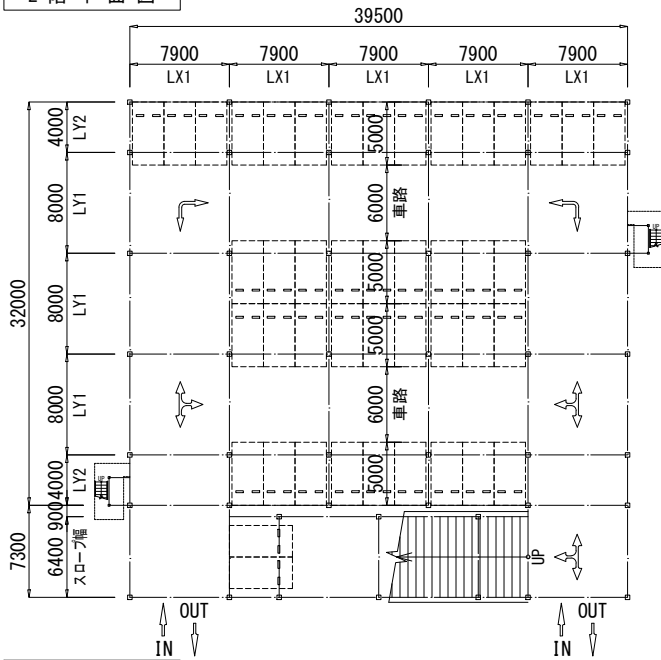
1階平面図
