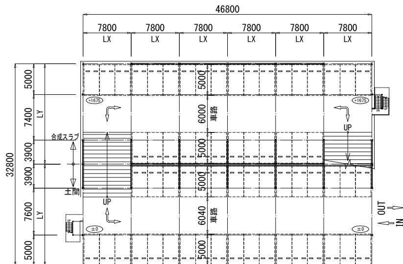
1階平面図
