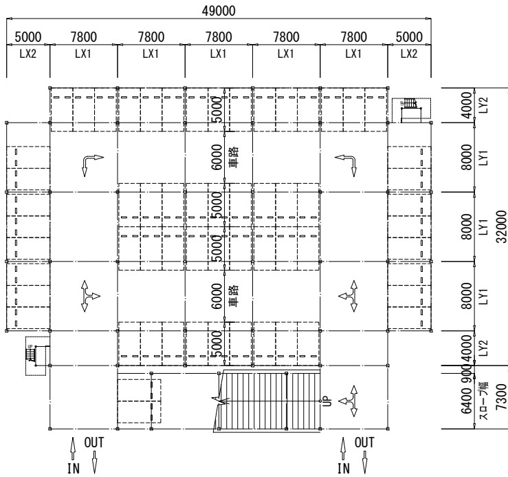
1階平面図
