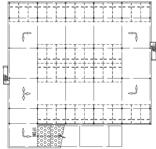
2階平面図
