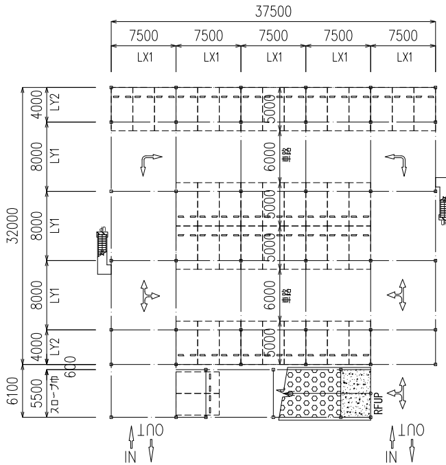
1階平面図
