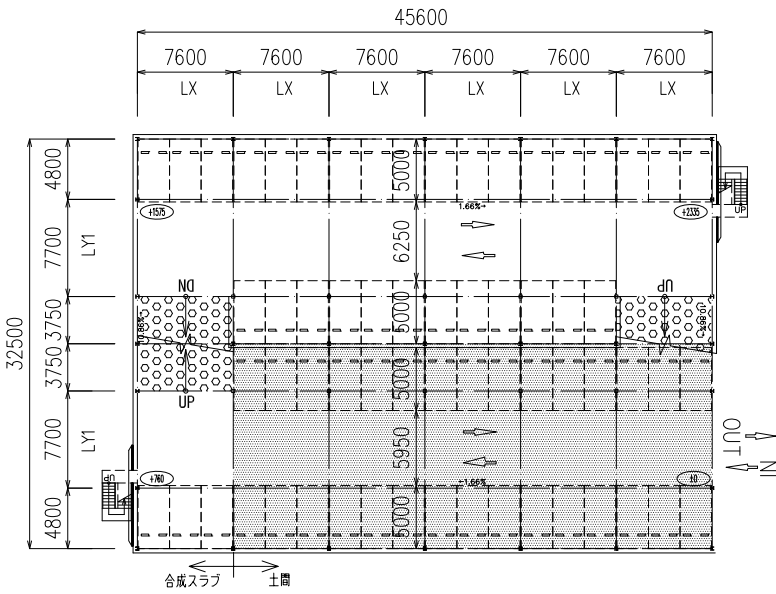
1階平面図
