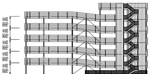
立面図
