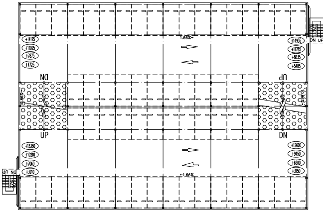
2~5階平面図
