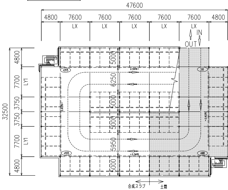
2~5階平面図
