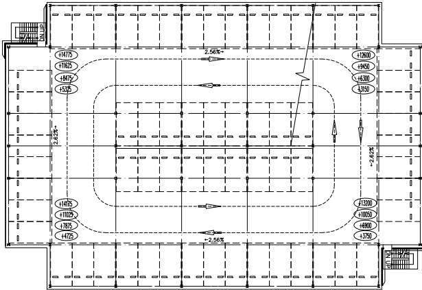
2~5階平面図
