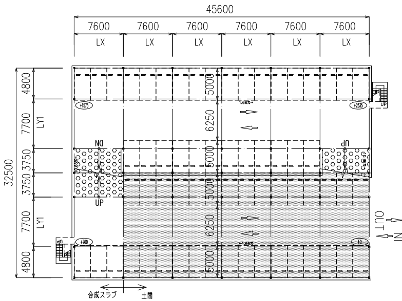
1階平面図
