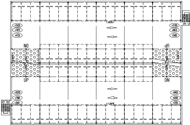
2~4階平面図
