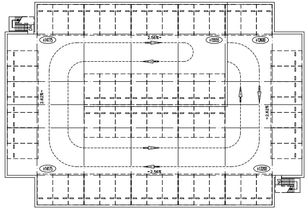
R階平面図
