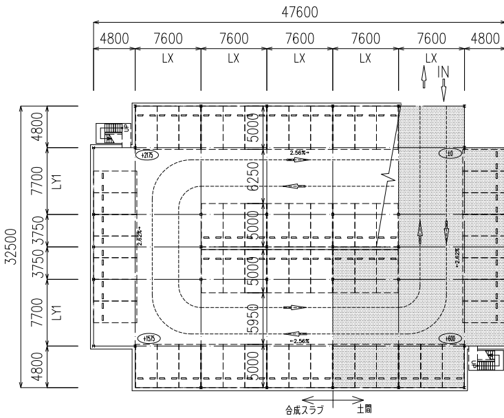
1階平面図
