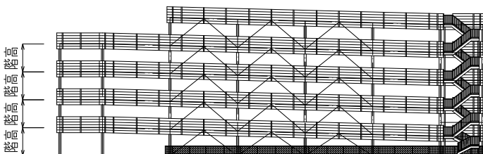
立面図
