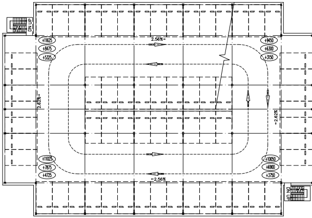
2~4階平面図
