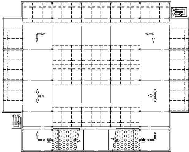
2~4階平面図
