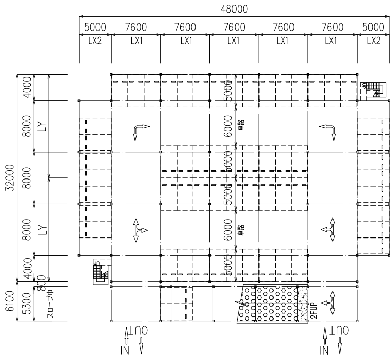
1階平面図
