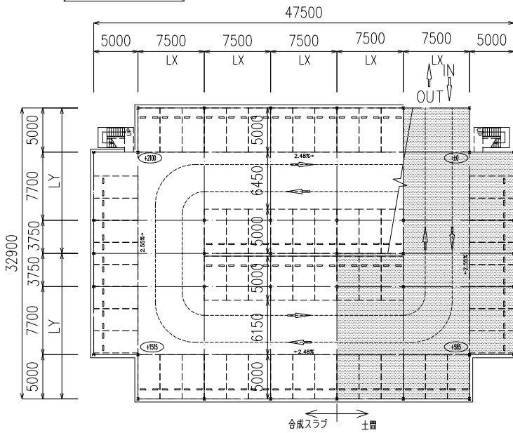
2~3階平面図
